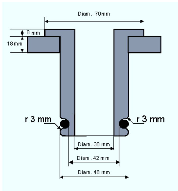
FIGURA 3. Sistema de suporte do preservativo
